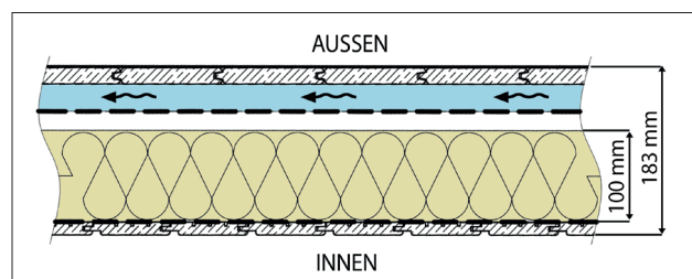
Abb.: Dachaufbau bei Gartensauna LUNA
