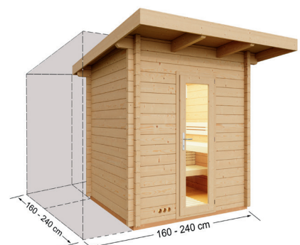
Abb.: Gartensauna TERRA - Optionen für Maßanfertigungen.
