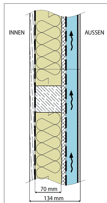
Abb.: Wandaufbau bei Gartensauna LUNA
