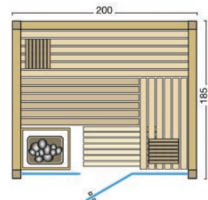
Abbildung Opal Massiv mit Sonderausstattung: Inneneinrichtung Fino, 2 VITALlight-IPX4-Strahler mit Easy Control-Steuerungen, Verdampferofen Hotline S8 und Steuerung Saunacontrol Xo in der Sauna montiert
