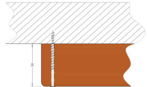
Sion 4 A - für Deckenmontage
